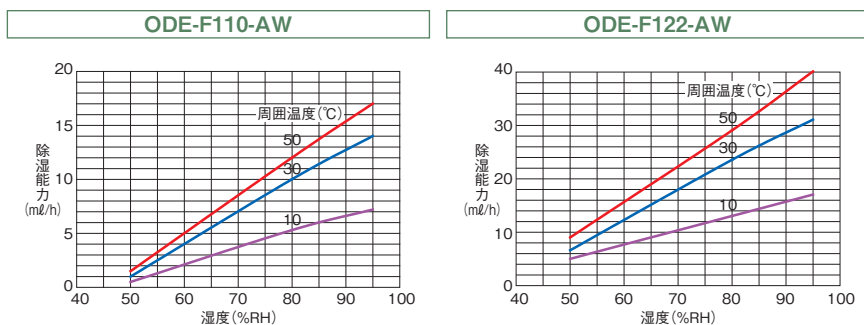
除湿特性表
