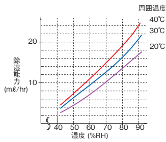
除湿特性表
